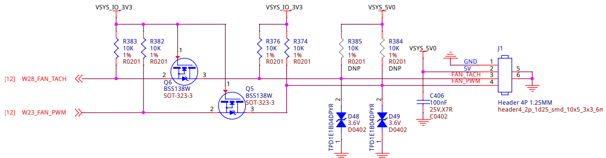
Fig. 3.23: Fan header
