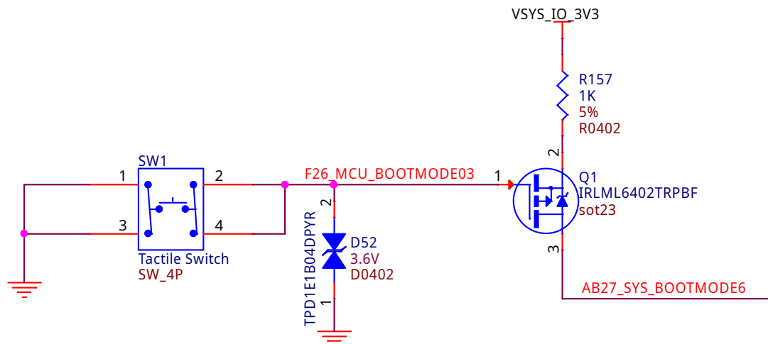
Fig. 3.30: Boot button
